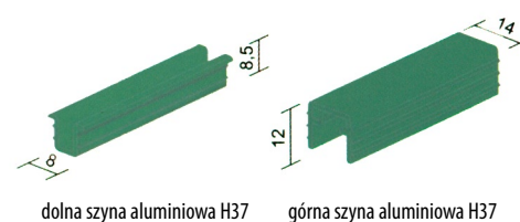
dolna szyna aluminiowa H37 górna szyna aluminiowa H37
