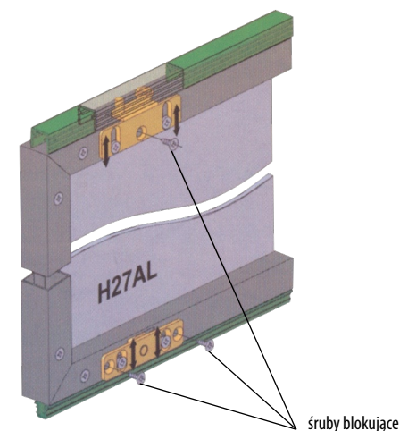
śruby blokujące
