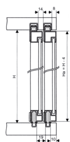
dolna szyna aluminiowa H37 górna szyna aluminiowa H37
